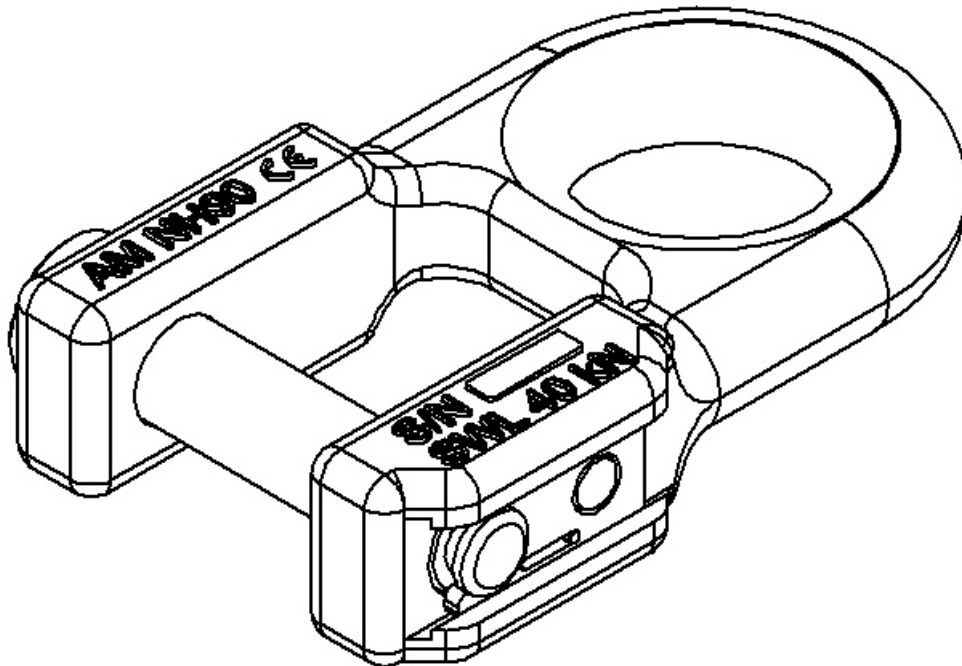
Fig.: Accessoire pour élingue P/N AM_NH90, certifié selon EN 1677-A1 (dimension 13), à utiliser avec les hélicoptères NH90 (annexe II) Développement: A&H ENG, Design Felix Muheim Formenbau Altdorf, Schmiedewerk pewag austria
